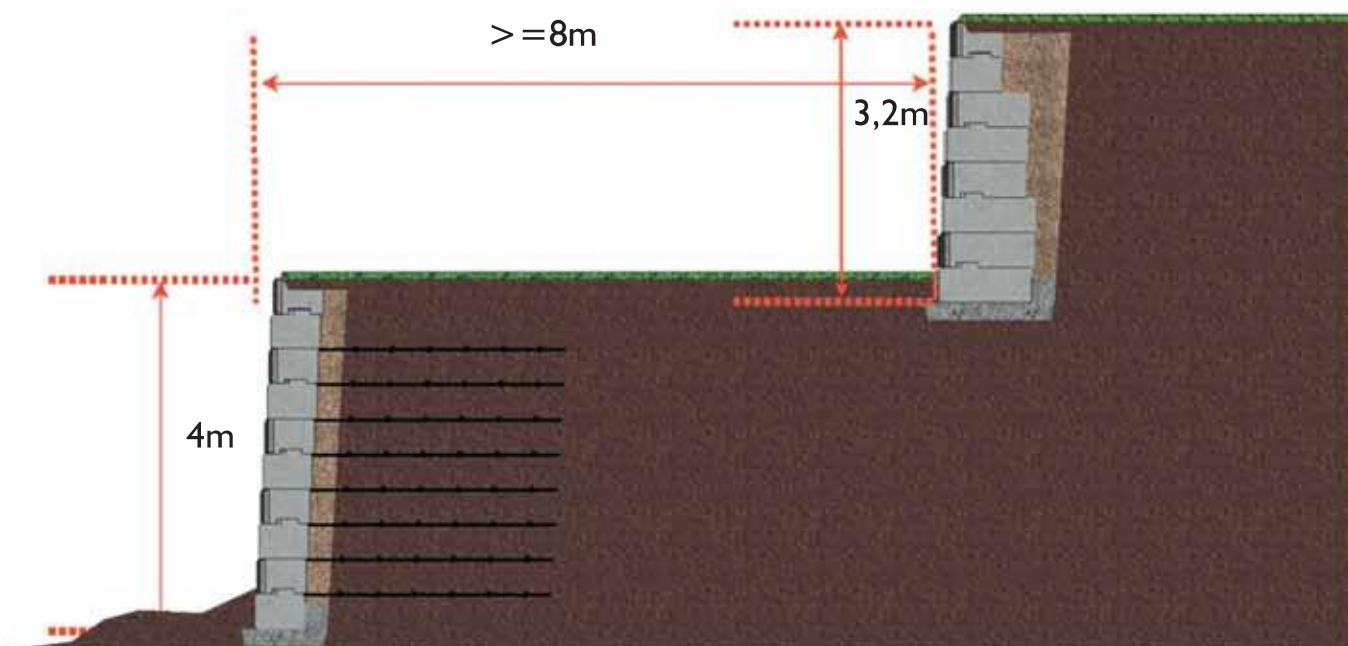
Eksempel på terrassemur
